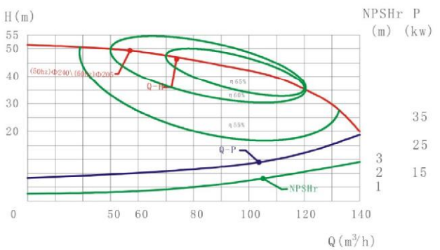
LX-40-2(Q-H曲线图/Graph)
