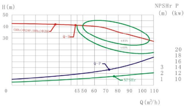
LX-40-1(Q-H曲线图/Graph)
