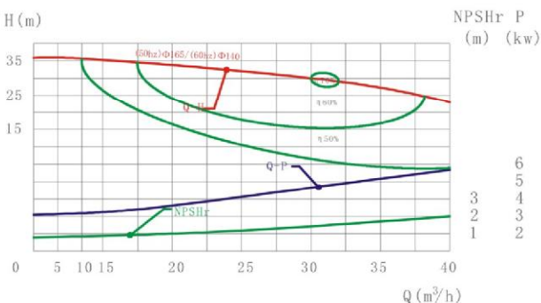
LX-20-1(Q-H曲线图/Graph)
