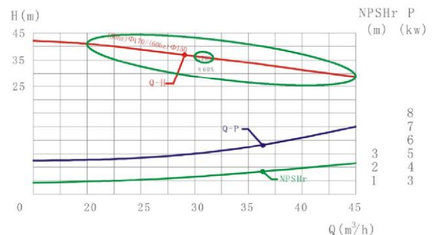
LX-20-2(Q-H曲线图/Graph)
