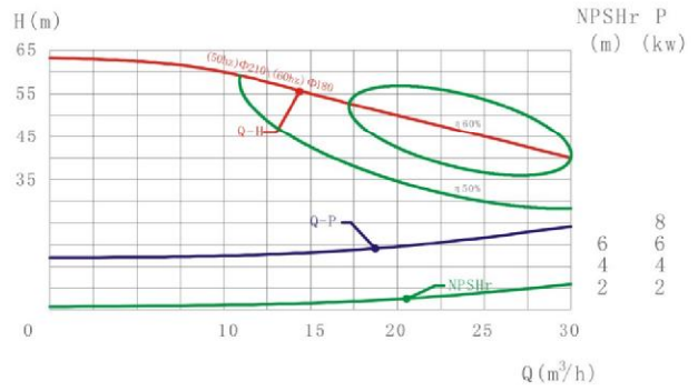
LX-35-2(Q-H曲线图/Graph)
