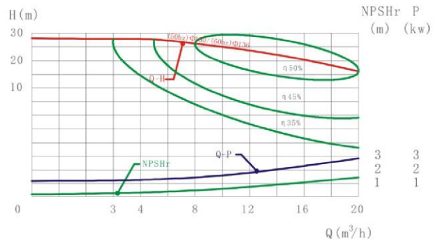
LX-15(Q-H曲线图/Graph)
