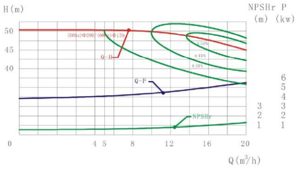
LX-35-1(Q-H曲线图/Graph)
