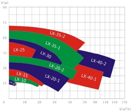
LX-10(Q-H曲线图/Graph)
