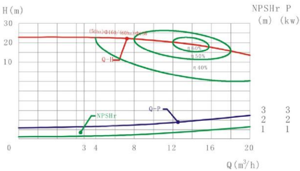
LX-10(Q-H曲线图/Graph)
