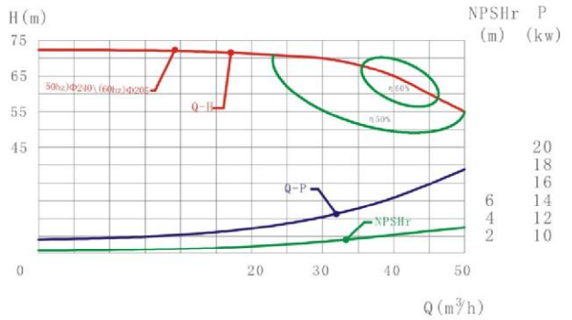
LX-35-2(Q-H曲线图/Graph)
